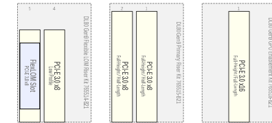
Riser
